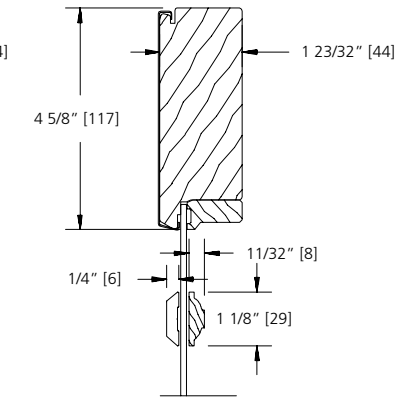
1 1/8" SDL BAR (PUTTY LINE)
