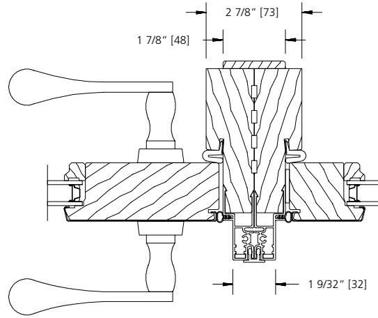
SIDE JAMB
