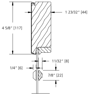
7/8" SDL BAR (PUTTY LINE)
